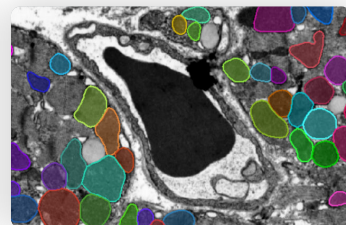
Mitochondria (TEM)
